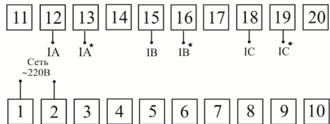
Рис. 8 – Клеммы подключения. Тип корпуса P99
