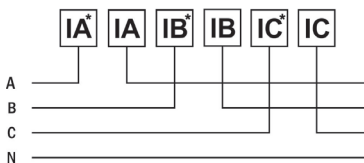
Рис. 9 – Подключение напрямую
