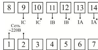
Рис. 7 – Клеммы подключения. Тип корпуса P77
